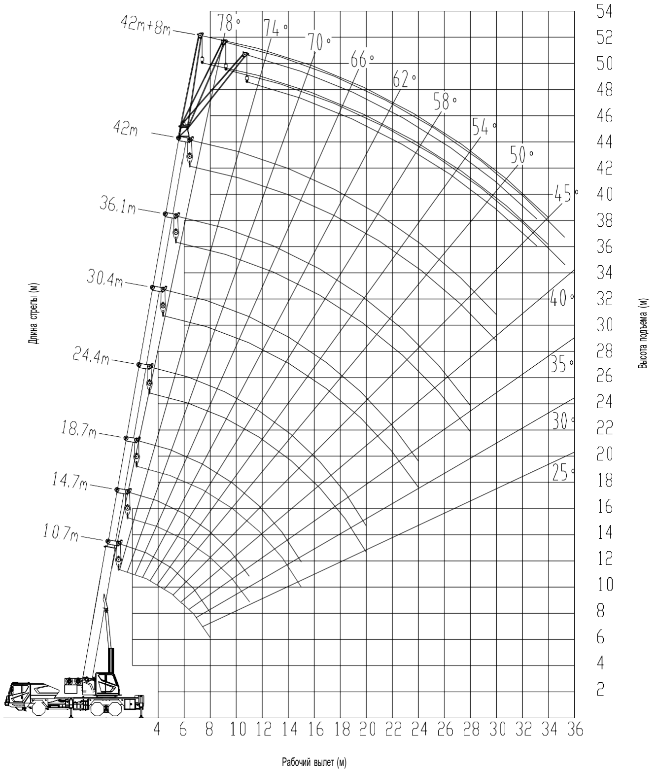
Рисунок 1 Грузовысотные характеристики
